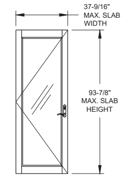
TYP. DOOR SLAB
